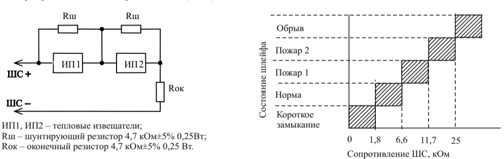
Рисунок 4 – Шлейф тепловых пожарных извещателей (тип 3)
